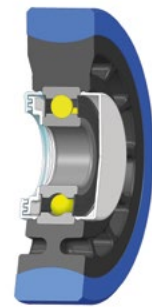
密封盖+单侧双密封 (CDS)
