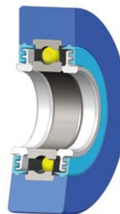
Rolle mit Doppeldichtung (2DS)
