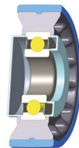
Rolle mit einseitigem Abdeckring und Deckel (CCR)
